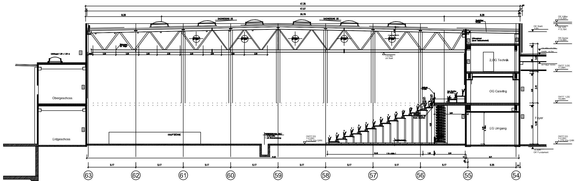
SCHNITT 62-62 (Achse g) Tribüne A ausgezogen
