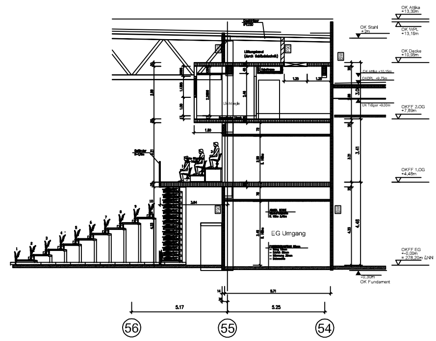
SCHNITT 64-64 (Achse h) Tribüne A teiltleskopiert
