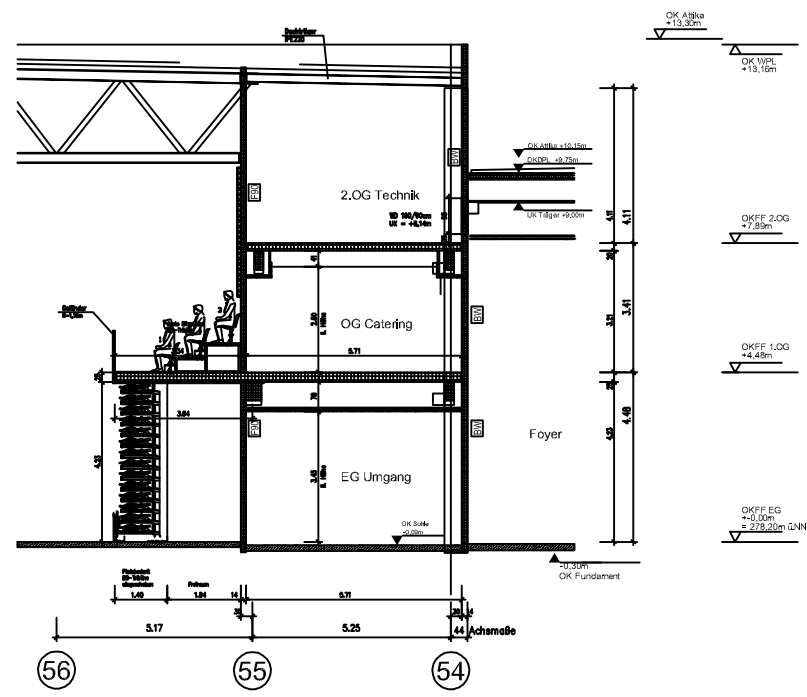
SCHNITT 65-65 (Achse k) Tribüne A eingeschoben
